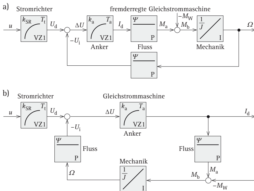
Bild 3.2 Strukturbild einer stromrichteragespeisten Gleichstrommaschine
