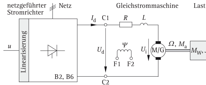
Bild 3.1 Stromrichtergespeiste Gleichstrommaschine
