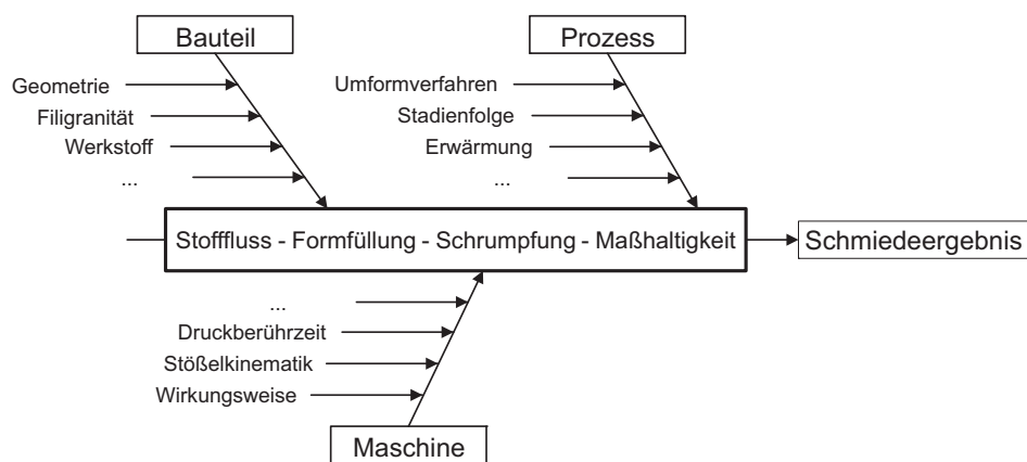
Abb. 2.5 Ishikawa-Diagramm mit Einflussgrößen auf das Schmedeergebnis
