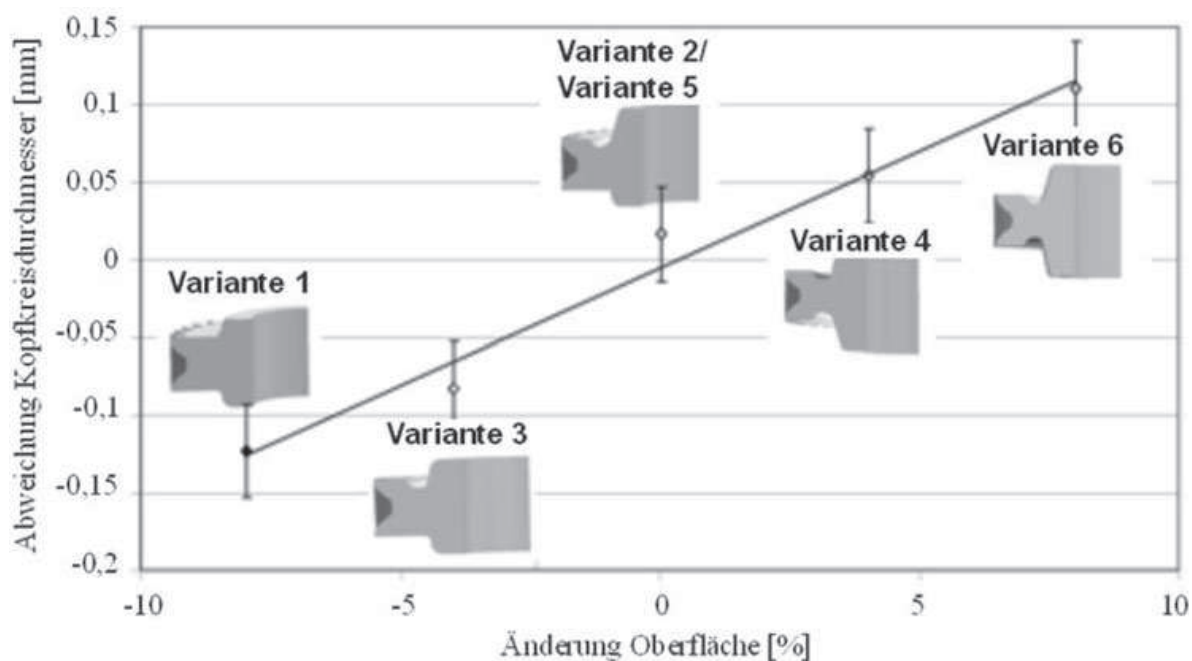
Abb. 2.6 Abhängigkeit des Kopfkreisdurchmessers von Grundkörpergestalt
