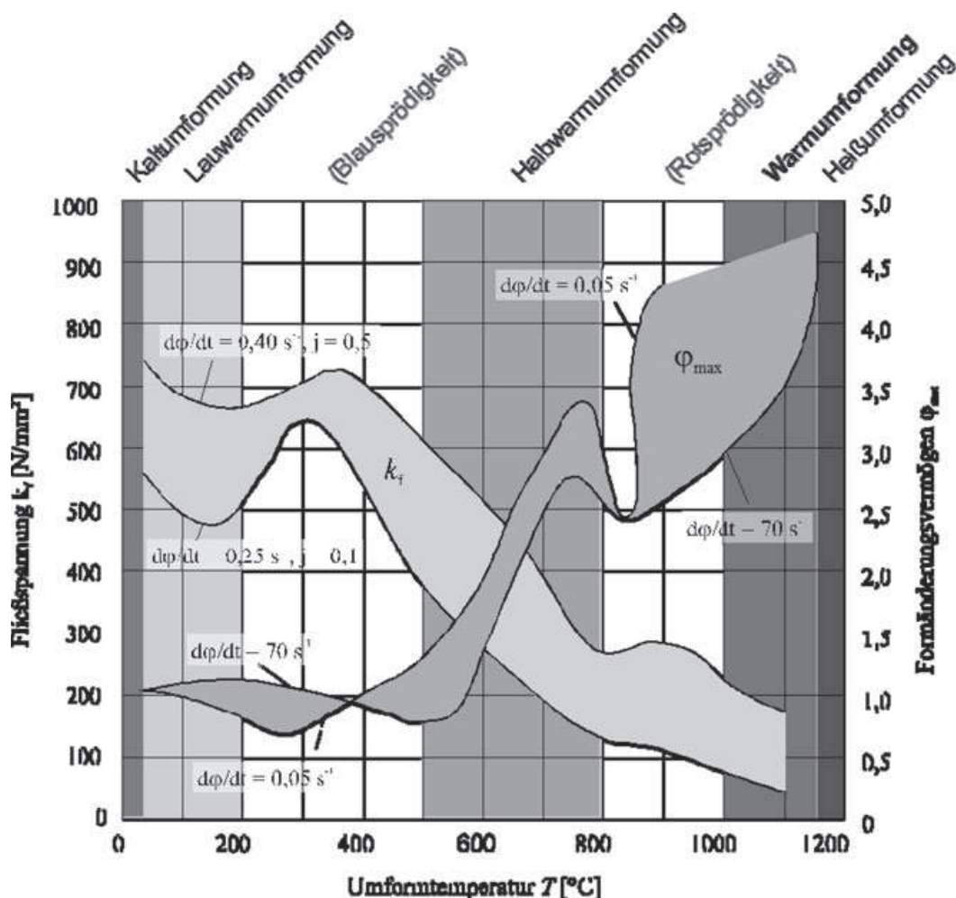
Abb. 2.2 Fließkurve/Formänderung über der Umformtemperatur von Schmiedestählen [Doe10]
