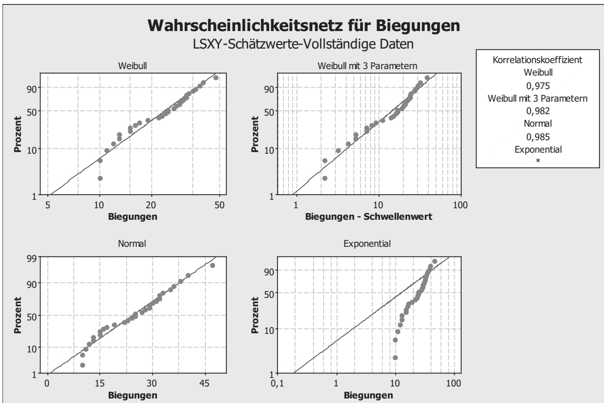
ABBILDUNG 6-15 Verteilungsidentifikation mit Minitab
