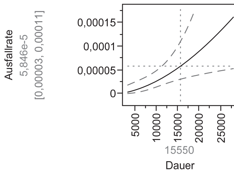
ABBILDUNG 6-19 Ausfallrate für die Ursache Material
