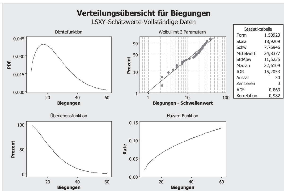
ABBILDUNG 6-16 Zuverlässigkeitsfunktion für die Lebensdauer der Büroklammern
