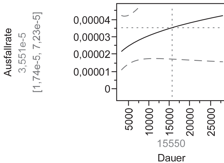
ABBILDUNG 6-18 Ausfallrate für die Ursache Getriebe
